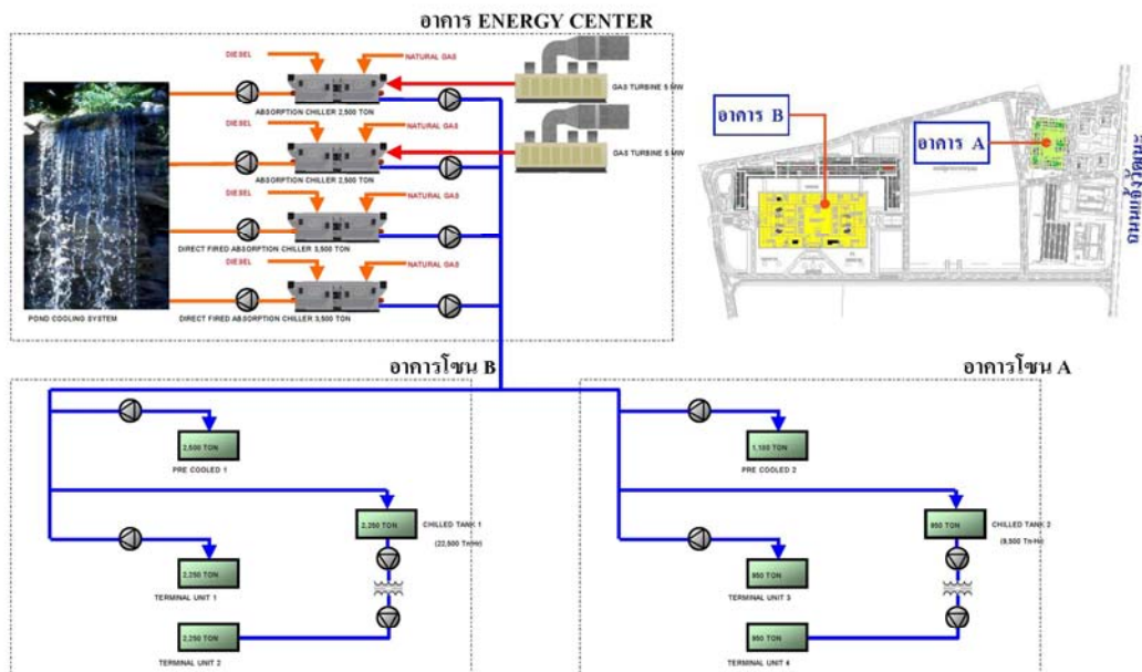
ไดอะแกรมระบบผลิตน้ำเย็นด้วยระบบ CO-GENERATION AND DISTRICT COOLING
